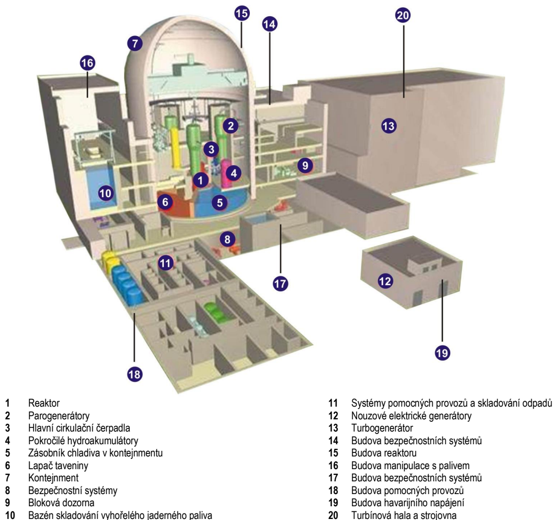
Obr. B.12: Ilustrativní řez elektrárenským blokem ATMEA1
