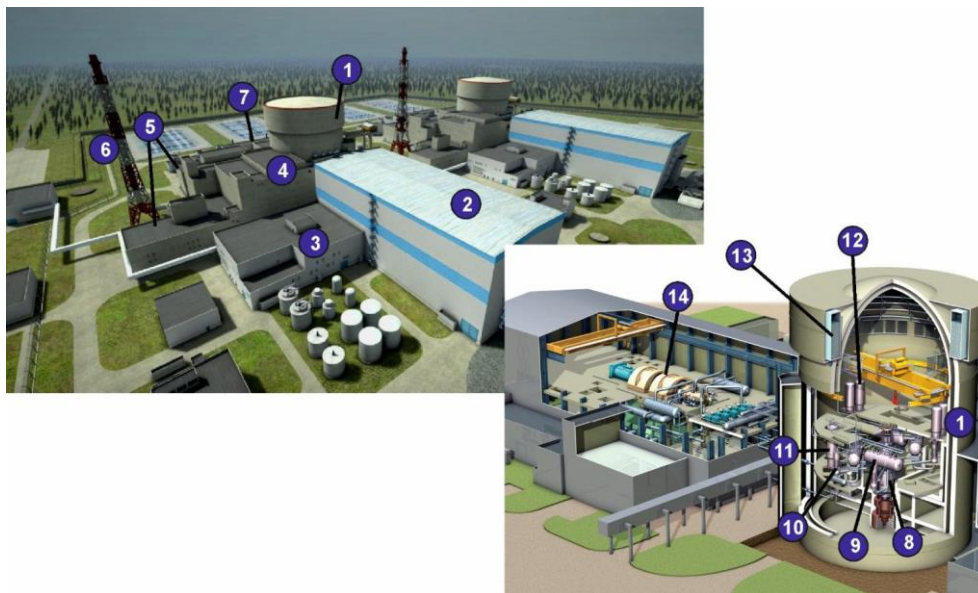
Obr. B.9: Ilustrativní řez elektrárenským blokem MIR-1200
