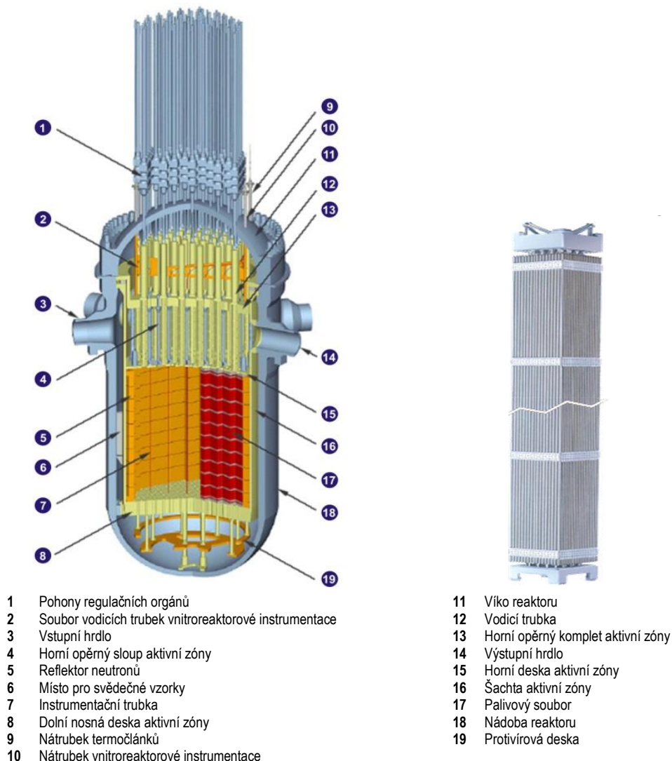
Obr. B.17: Typické konstrukční řešení reaktoru typu PWR, příklad řešení palivového souboru
