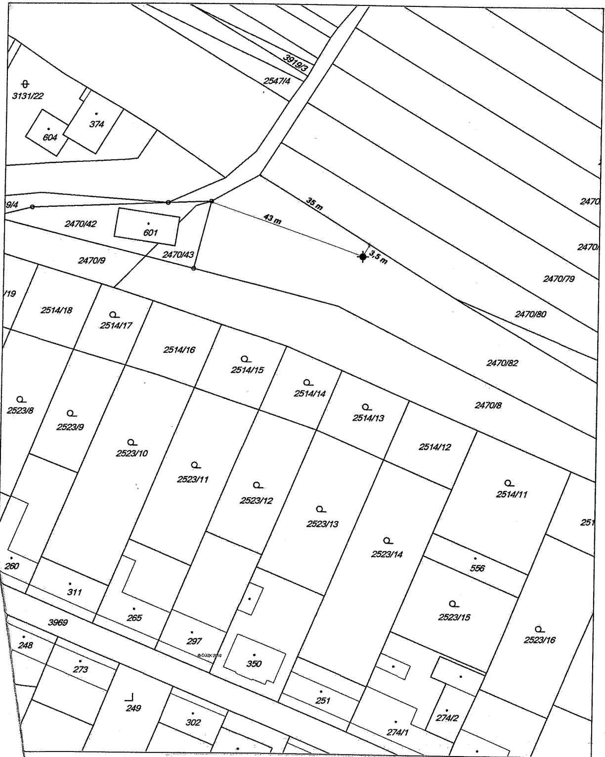
Příloha 1: Zákres projektované studny na parc. č. 2470/82 v kat. úz. Višňové (1 : 1 000)
